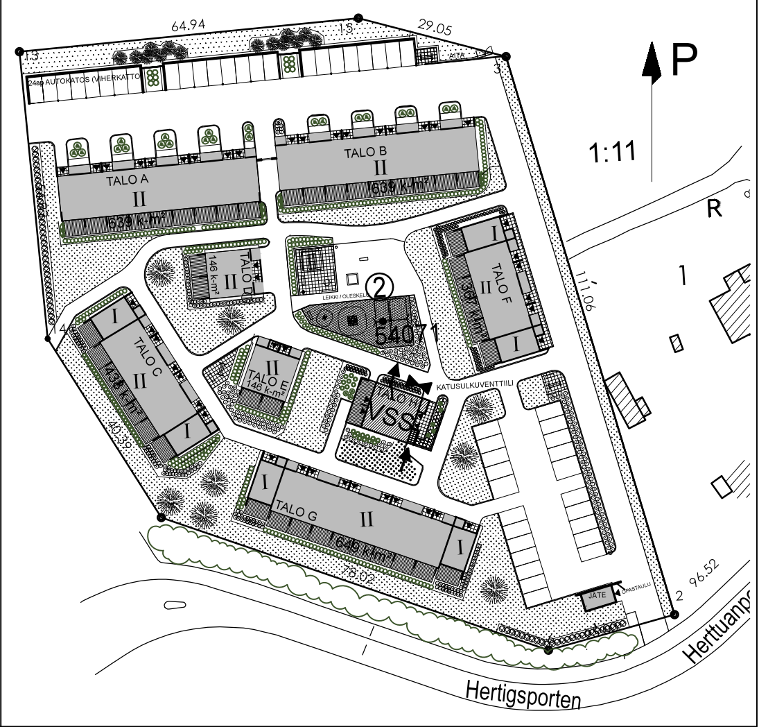
ASEMAPIIRUSTUS 1:1000
