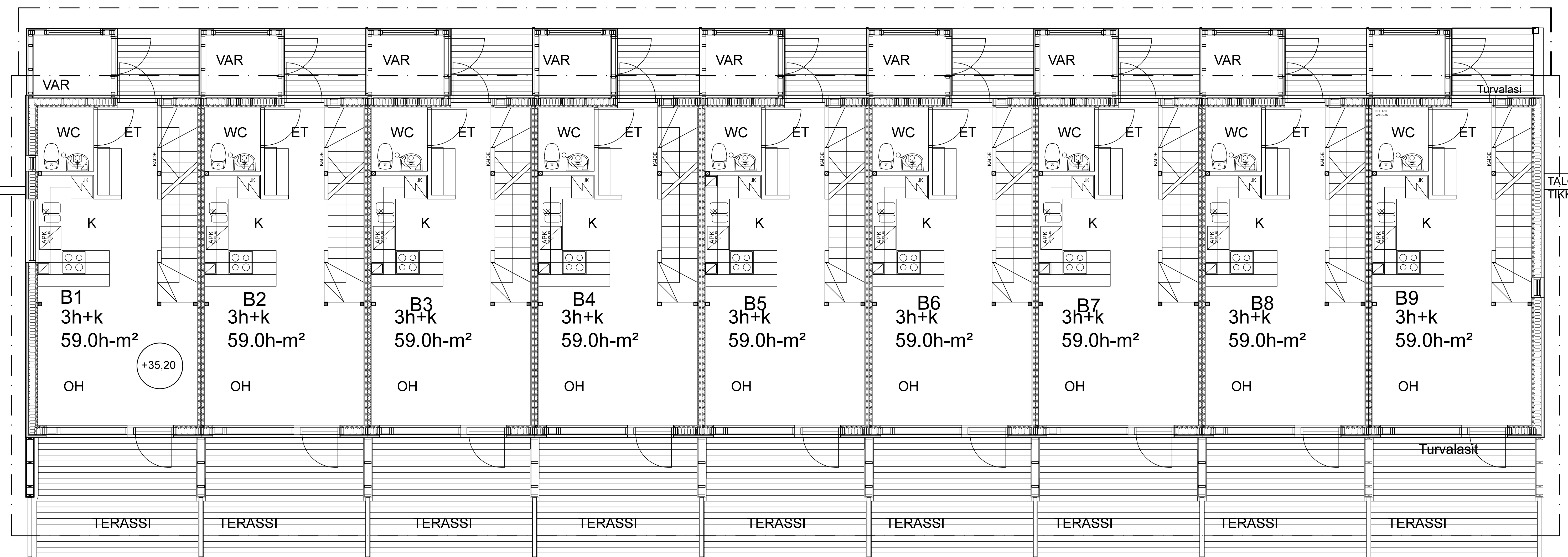
TALO B, 1KRS, lattiakorko +35.20
